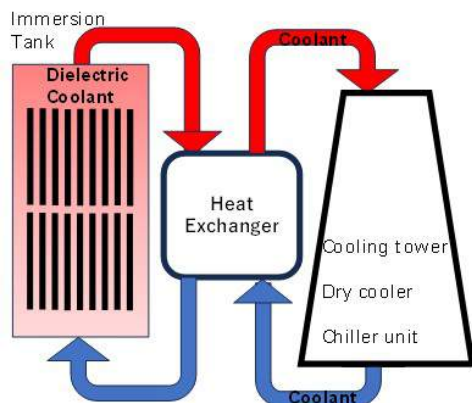
図 1 浸透冷却システムの概略
