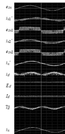
図 2 各部の波形
