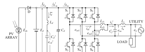
図 1 単相複合 PWM 電圧形インバータ
