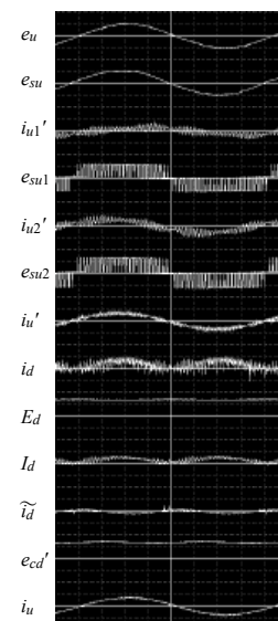
図 2 各部の波形
