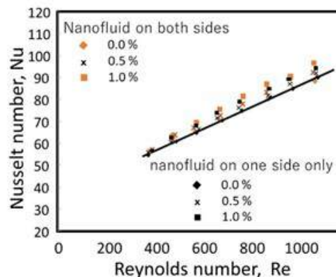
図 2 異なった作動媒体の冷却性能
