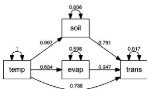
図 1: パス解析
